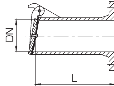
Fig. 125 mit Flanschsanschluss PN 10/16
