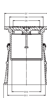
Schnitt A-A
