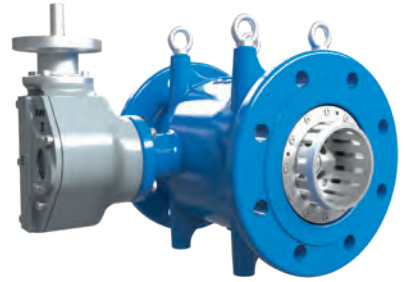
mit Schlitzzylinder
