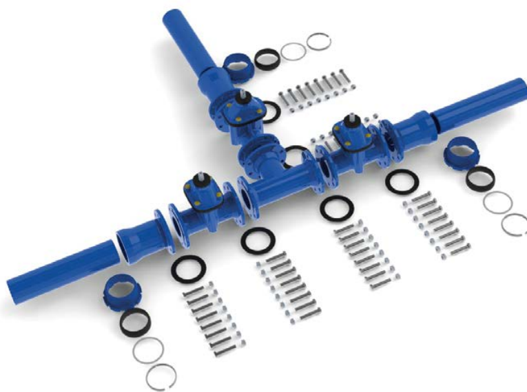
Der gleiche Aufbau mit Flanschverbindungen und 124 Montageteilen
